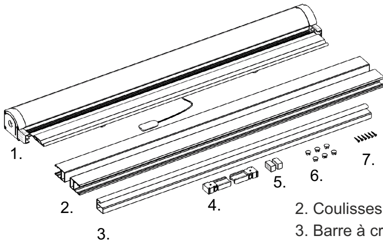
1. Moustiquaire. 4. Raccords de coulisses. 7. Vis.
