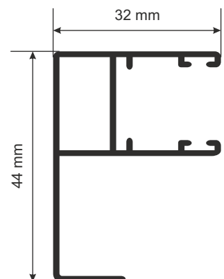
Fig. 3 Coulisse déportée. (en option)
