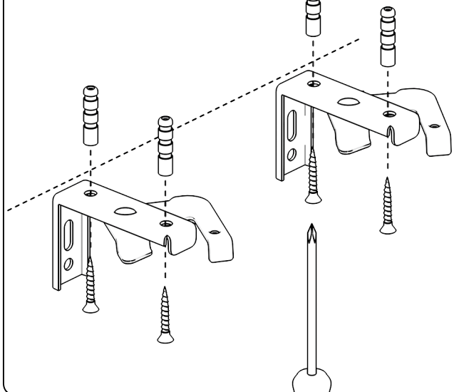
Montage des supports – au plafond.
