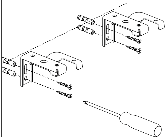
Montage des supports – au mur.
