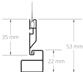
Hauteur de la barre inférieure et de la barre à crochet.
