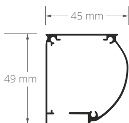
Dimensions du caisson.
